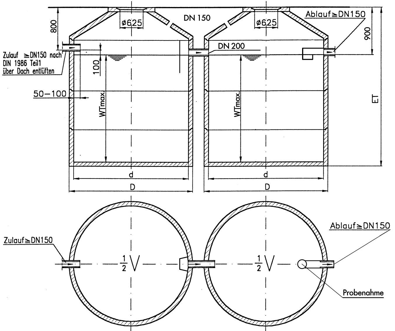
Maßtabelle für Schmitgen-Zweikammer-Kleinkläranlagen, Zn. SBR D 12-20
